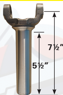
Part# FTSFS005
