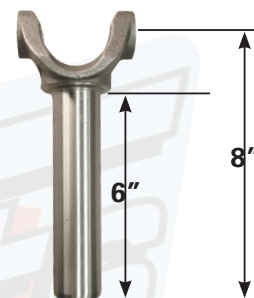
Part# FTSFS006
